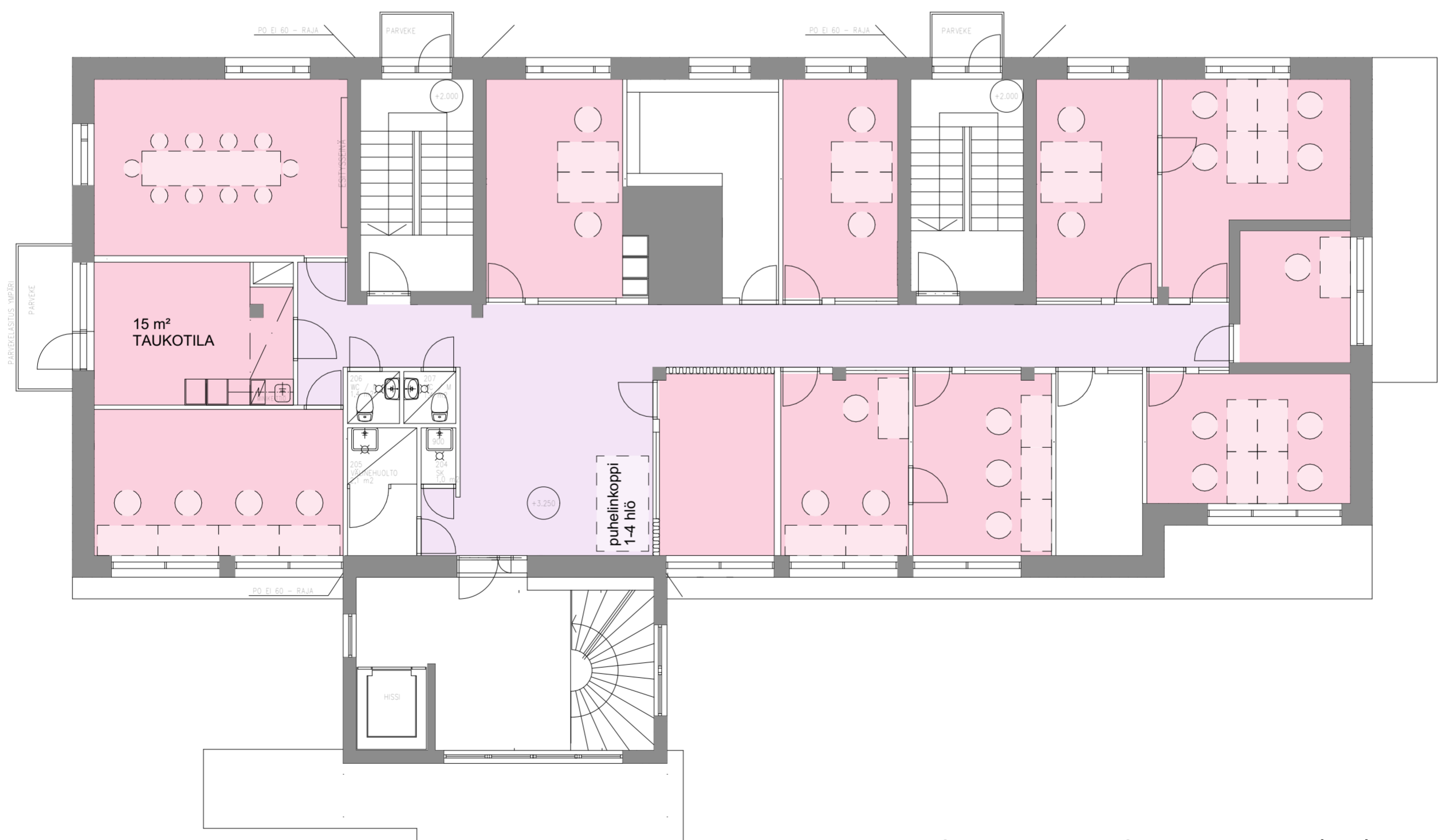
Pohjapiirros, 2. kerros, 1:100 (A2)
