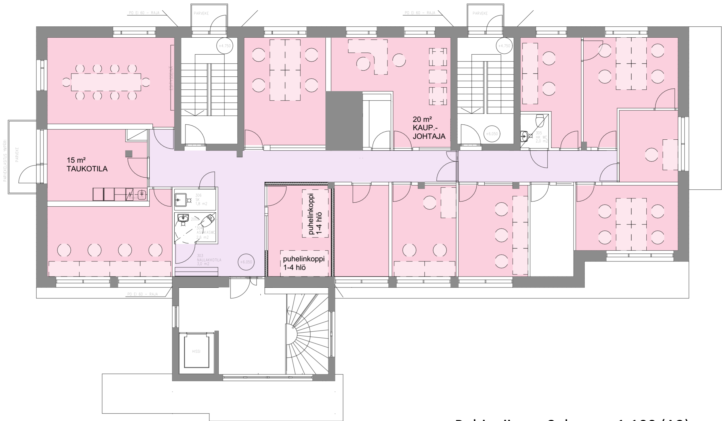
Pohjapiirros, 3. kerros, 1:100 (A2)
