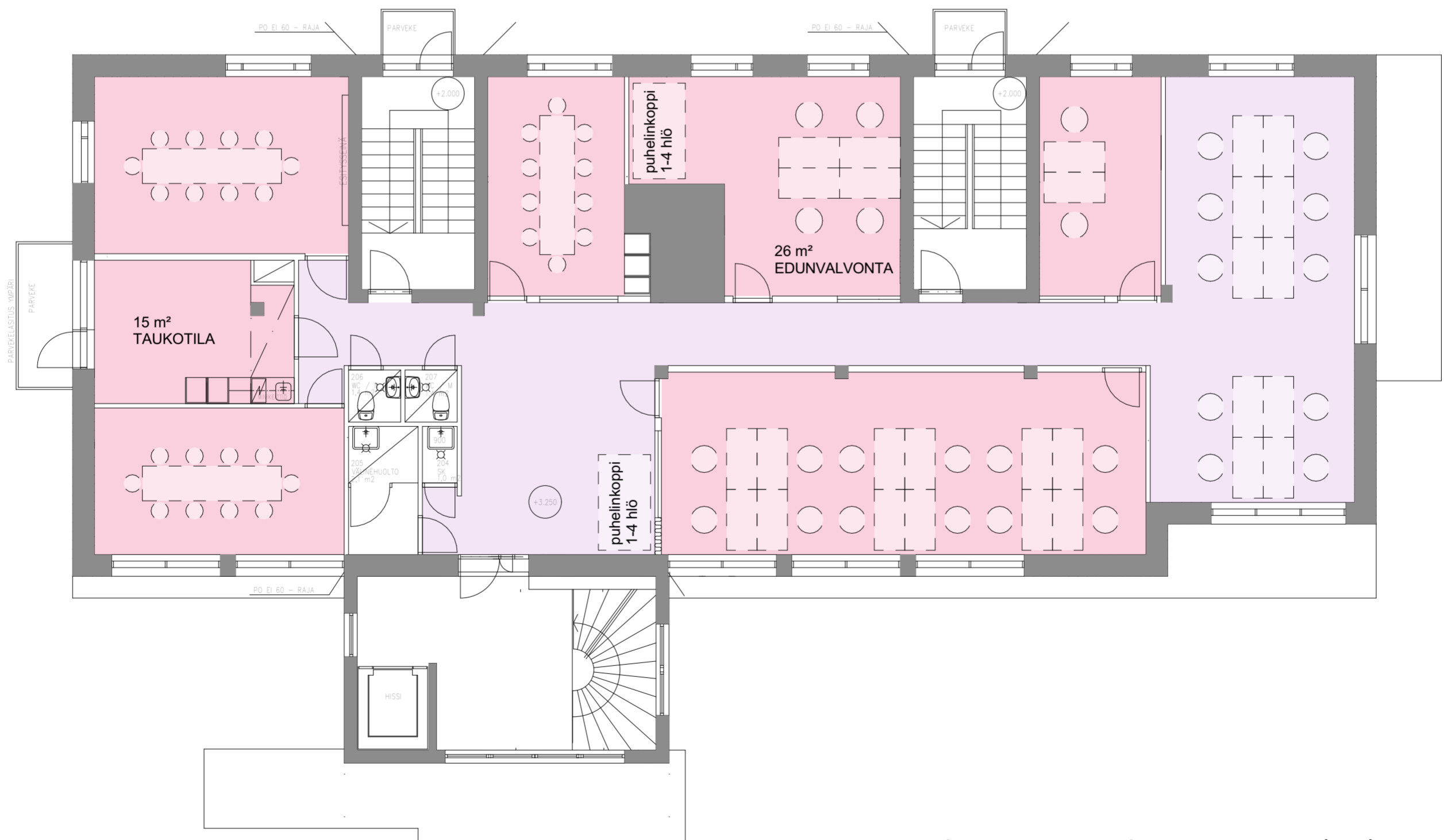
Pohjapiirros, 2. kerros, 1:100 (A2)
