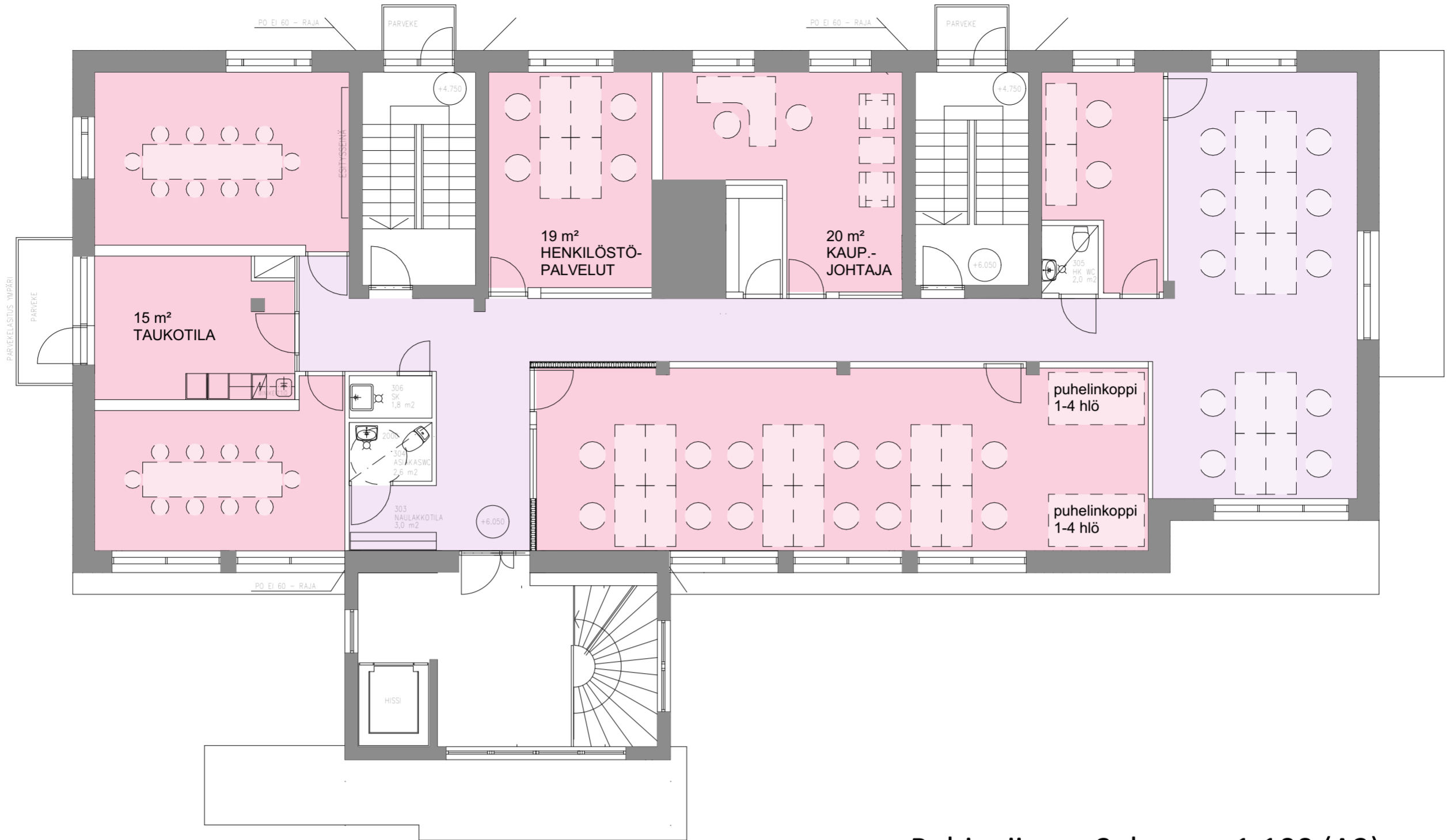
Pohjapiirros, 3. kerros, 1:100 (A2)
